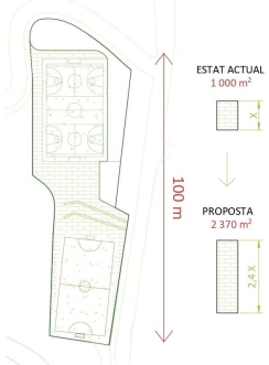
PLANTA COBERTA PISTA I PLANTA BAIXA EDIFICIS E: 1/400
