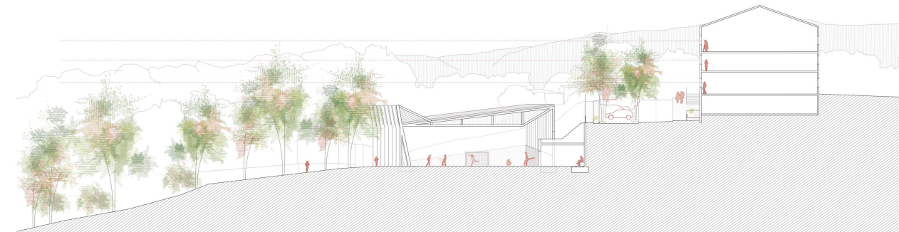
SECCIÓ TRANSVERSAL - TRAM INFERIOR E: 1/300
