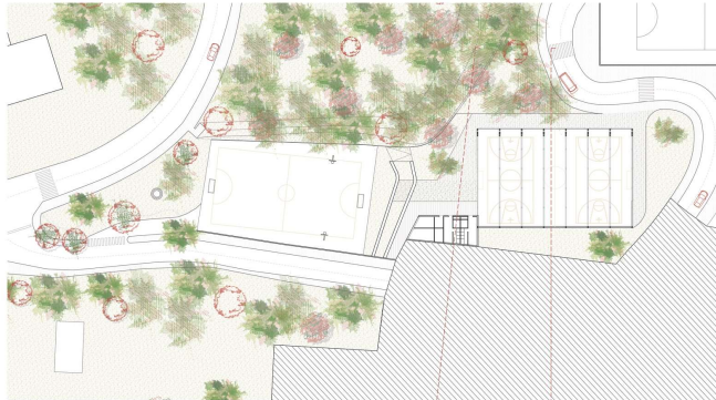
PLANTA PISTA I PLAÇA - NOU ESPAI POLIVALENT
